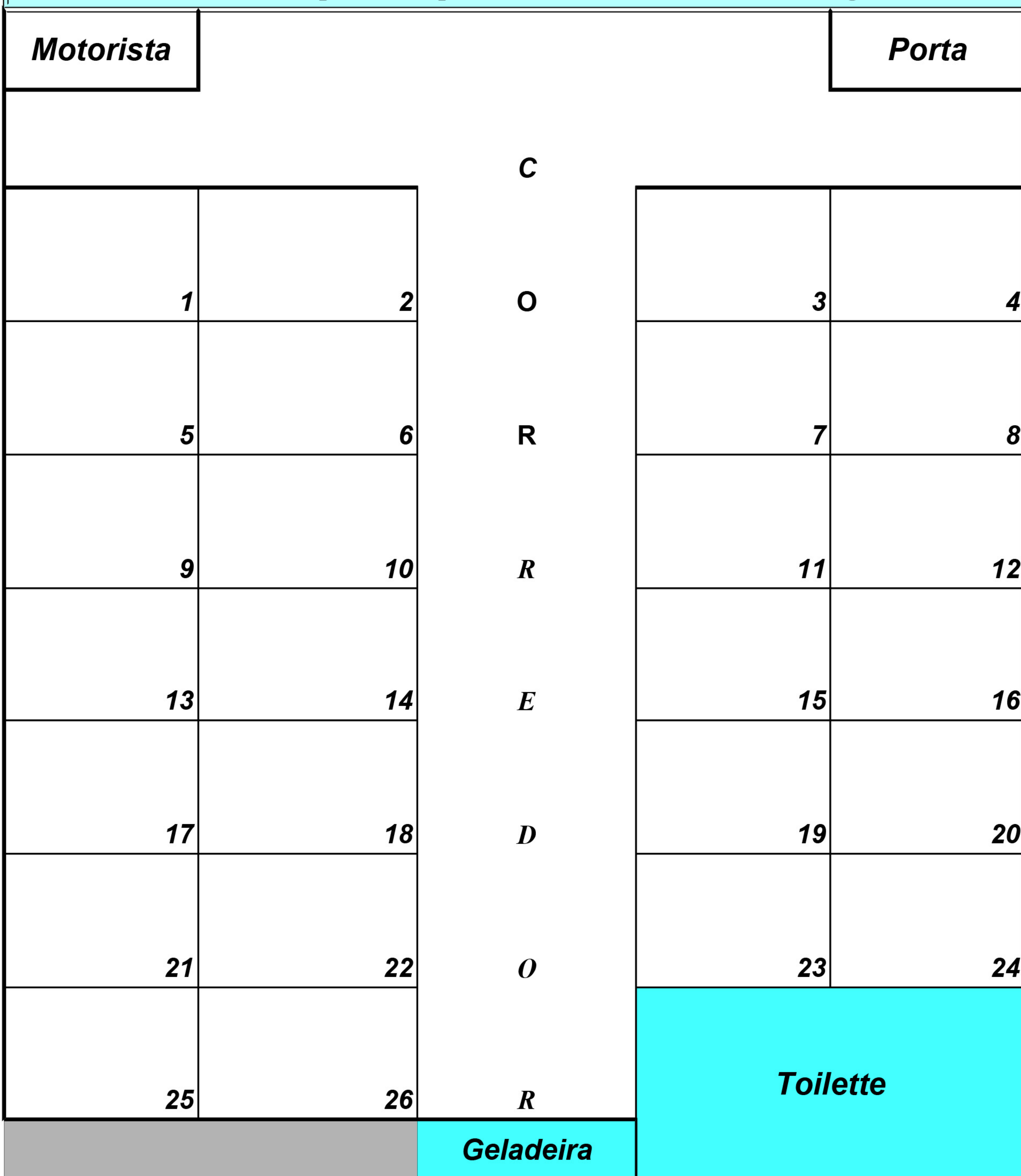
Esquema das poltronas >>Micro-ônibus com 26 lugares
